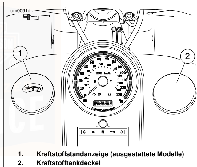
Abbildung 25. Kraftstofftank
