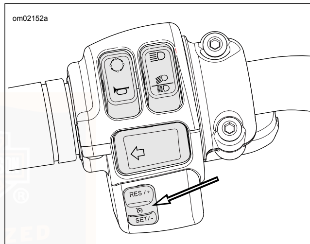
Abbildung 5. Geschwindigkeitsregelung: FLSS, FLSTC, FLSTFBS, FLSTN
