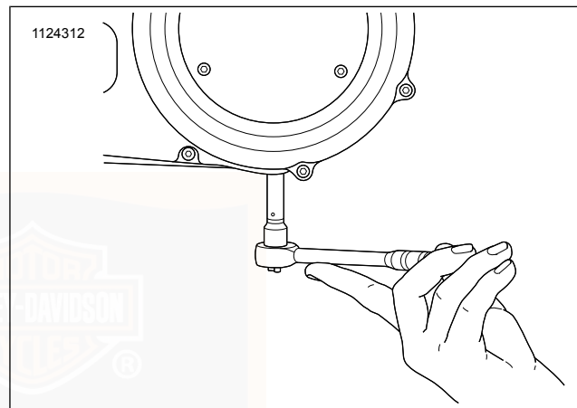
Abbildung 46. Ausbau/Einbau der Kettengehäuse-Ablassschraube
