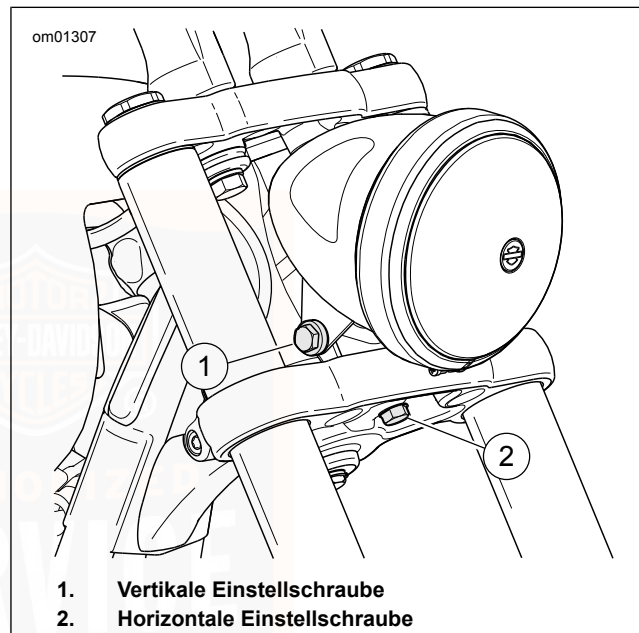
Abbildung 60. Scheinwerfereinstellung (typisch)
