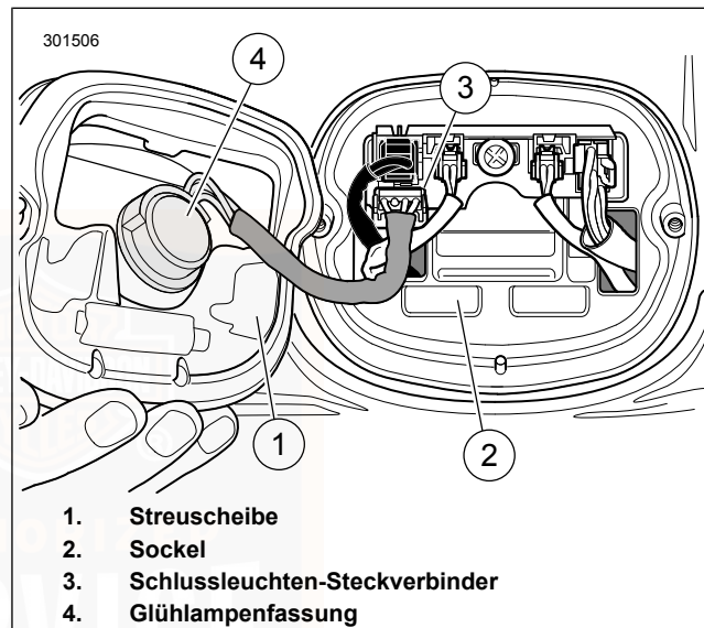
Abbildung 63. Schlussleuchtenbaugruppe
