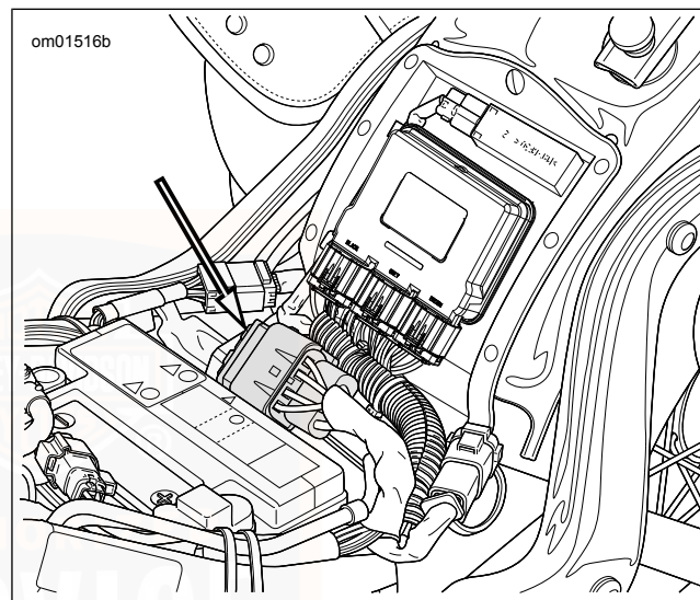
Abbildung 75. Lage des Sicherungsblocks
