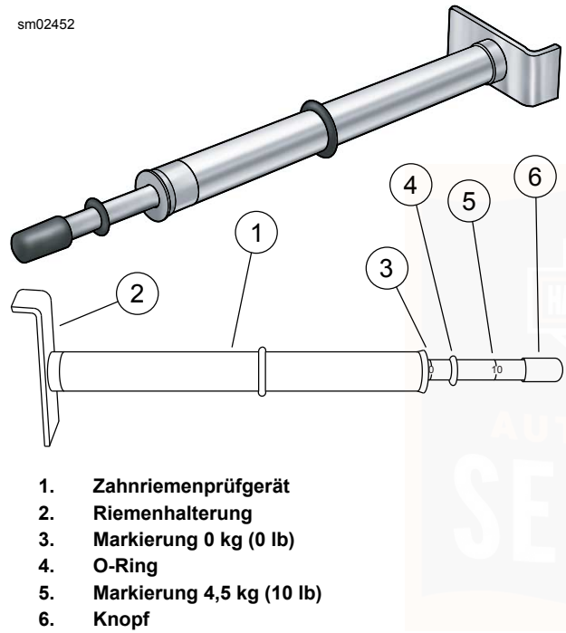
Abbildung 49. Zahnriemenprüfgerät
