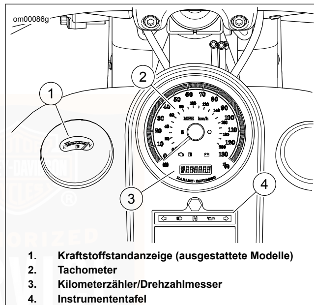
Abbildung 13. Instrumente: Alle außer FXSB
