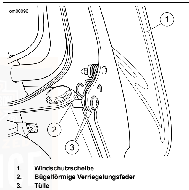
Abbildung 32. Windschutzscheiben-Baugruppe
