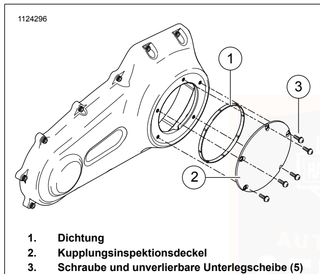
Abbildung 47. Kupplungsdeckel (Typisch)
