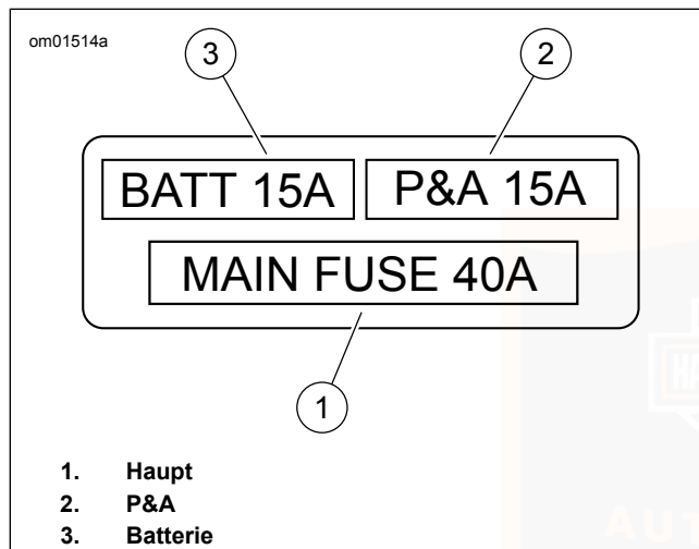
Abbildung 74. Sicherungsblock
