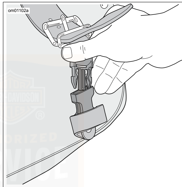
Abbildung 30. Satteltaschen-Schnelllösevorrichtung
