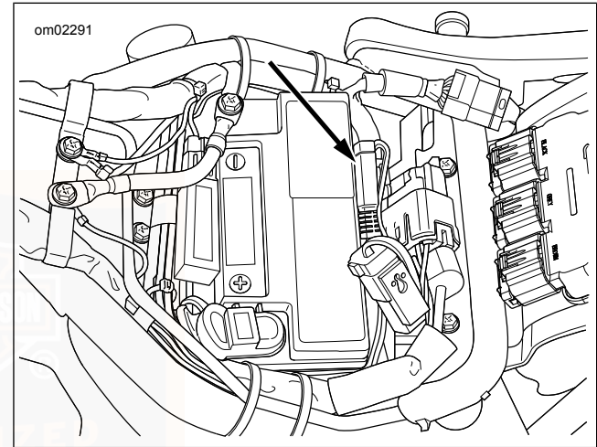
Abbildung 69. Batterieladegerät-Steckverbinder (typisch)
