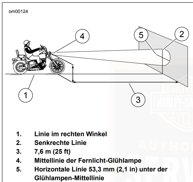
Abbildung 58. Scheinwerferausrichtung
