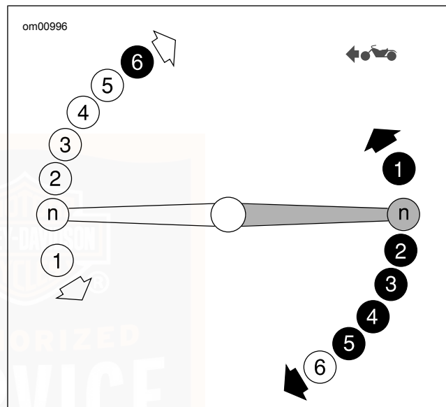
Abbildung 22. Fersen-/Fußspitzenschalthebel
