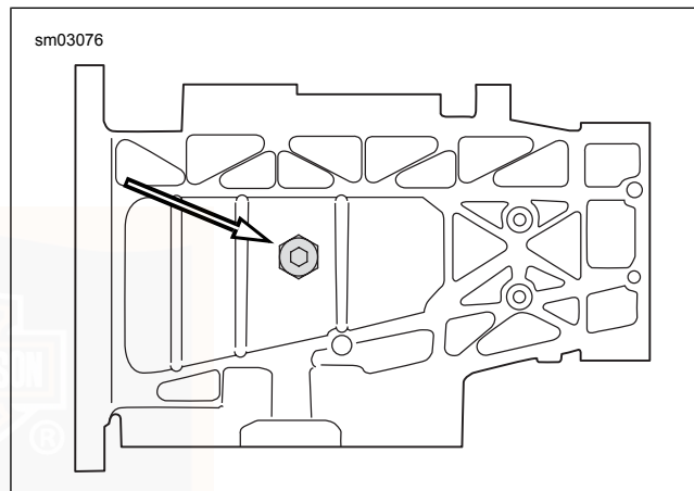
Abbildung 45. Getriebschmiermittel-Ablassschraube (Ansicht von unten)
