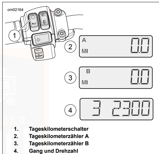
Abbildung 15. Tageskilometerzähler, Drehzahlmesser/Ganganzeige
