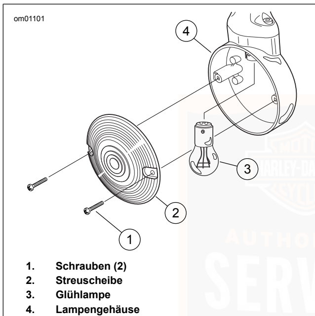
Abbildung 62. Blinker-Baugruppe: Flachglasausführung
