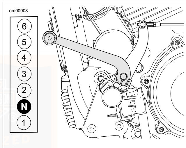
Abbildung 21. Schalthebel und Schaltmuster FERSEN-/FUßSPITZENSCHALTHEBEL
