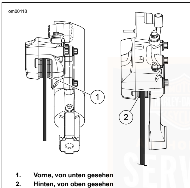
Abbildung 51. Bremsbelagmaterial
