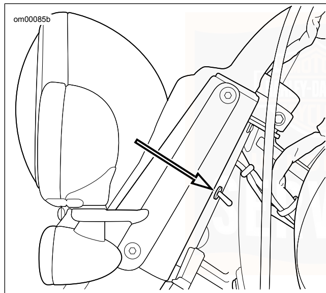
Abbildung 28. Zusatz-/Nebelscheinwerferschalter
