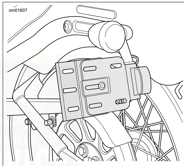
Abbildung 27. Seitlich befestigte Kennzeichenbaugruppe ZUSATZ-/NEBELSCHEINWERFER: FLSTC, FLSTN
