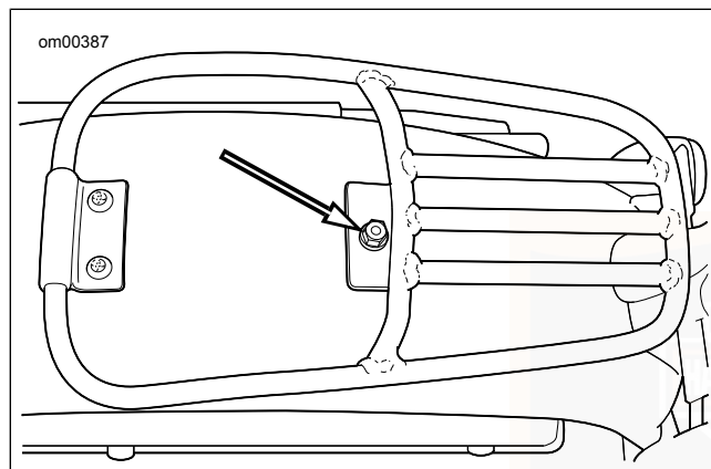
Abbildung 79. Sitzbefestigungsbolzen: FLSTN SITZE: FLS, FLSS
