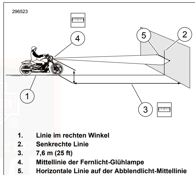
Abbildung 59. LED-Scheinwerferausrichtung SCHEINWERFEREINSTELLUNG
