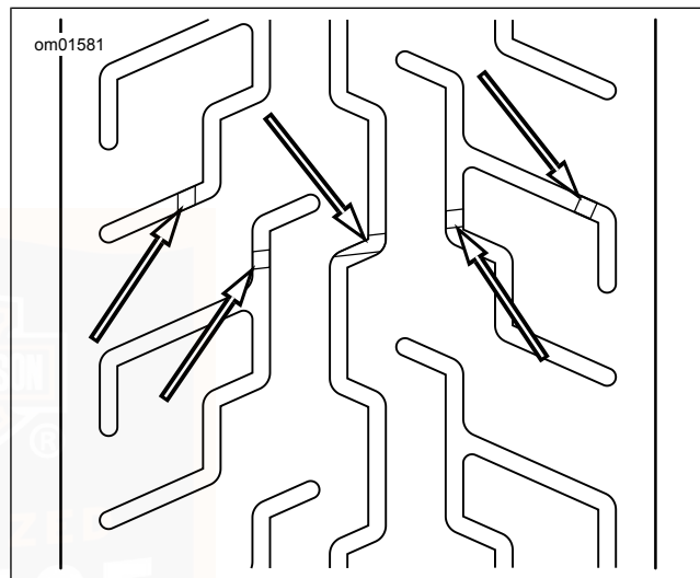
Abbildung 53. Dunlop-Reifen, Aussehen der Profilverschleißanzeigen
