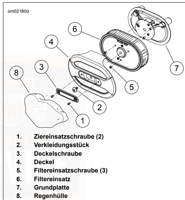
Abbildung 54. Luftfilter: FLSTFBS
