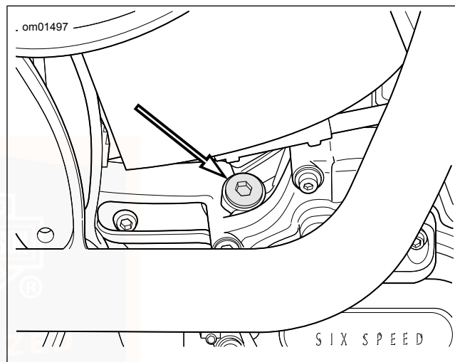
Abbildung 43. Lage des Getriebeeinfüllverschlussstopfens/Ölmesstabs
