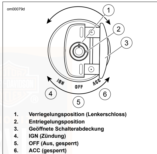
Abbildung 12. Zündschalter: Alle außer FXSB
