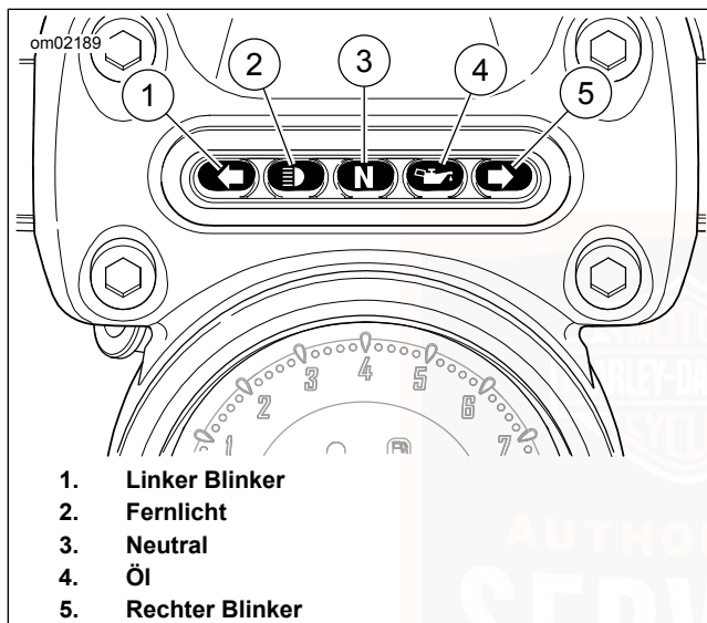
Abbildung 16. Kontrollleuchten
