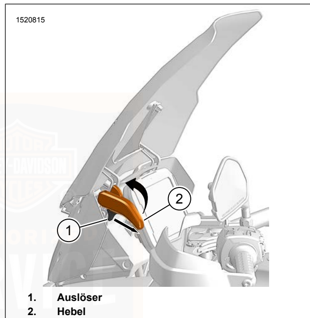
Abbildung 49. Höheneinstellung Windschutzscheibe
