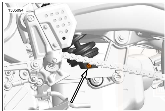
Abbildung 15. Zugstufeneinsteller
