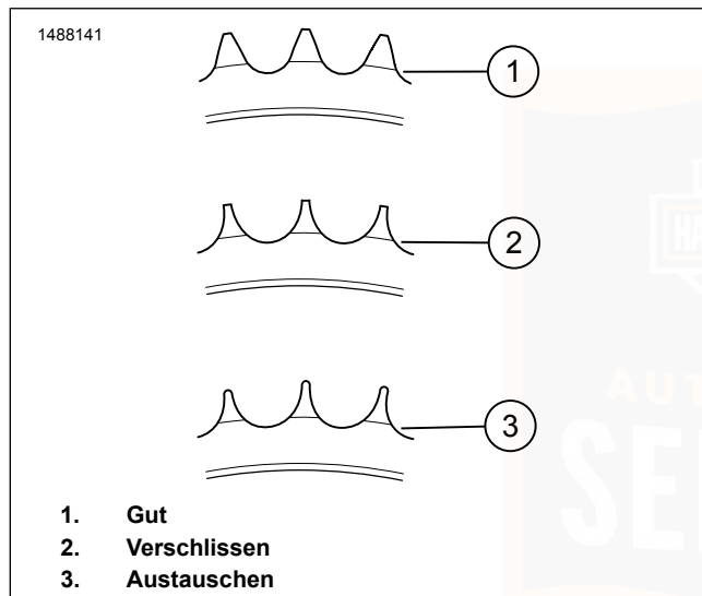
Abbildung 60. Zahnradzahnzustand
