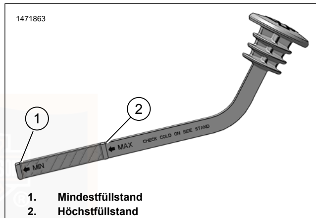
Abbildung 63. Kühlmittel-Einfüllverschlussstopfen/Messstab
