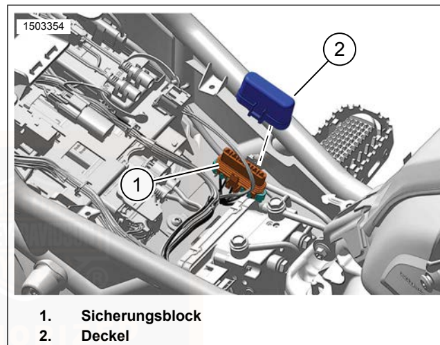
Abbildung 85. Sicherungsblock – Lage
