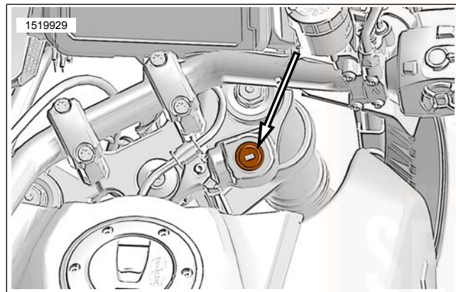
Abbildung 30. Gabelschloss
