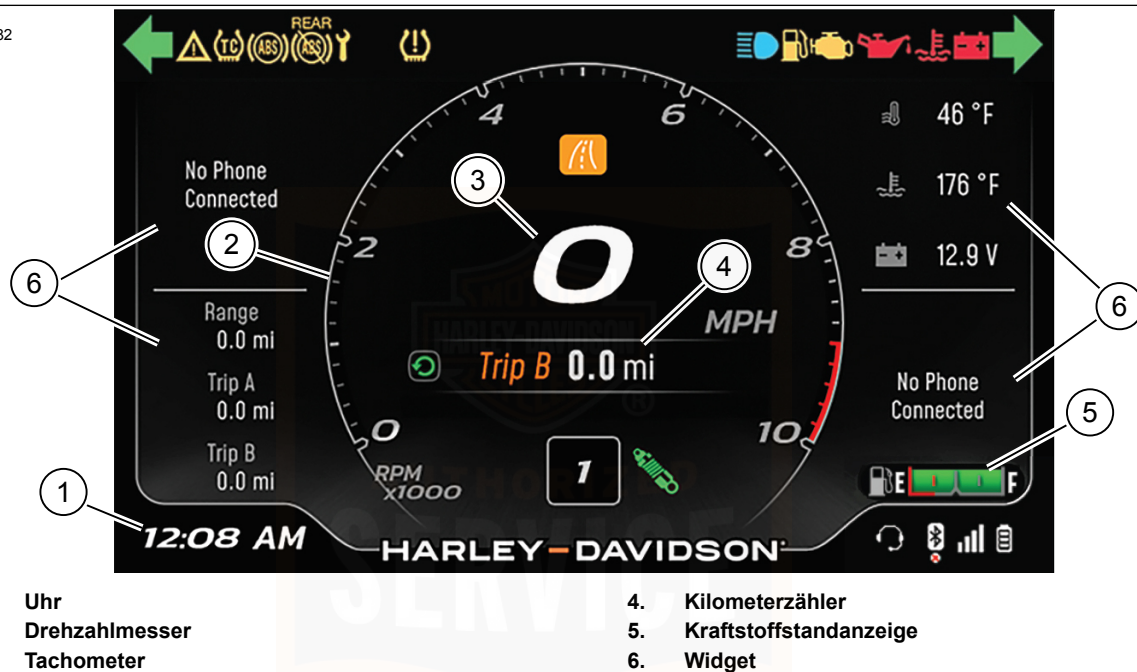
Abbildung 31. Instrumente: Dashboard-Anzeige
