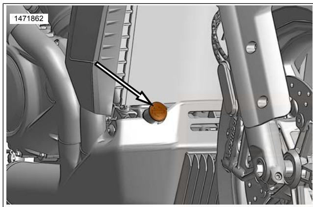
Abbildung 62. Kühlmittel-Einfüllverschlussstopfen/Messstab
