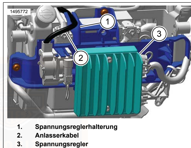
Abbildung 70. Negative Kabelhalterung
