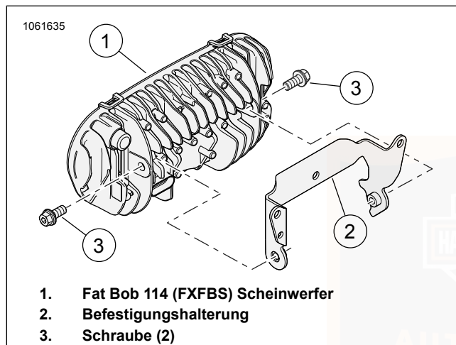
Abbildung 80. Scheinwerfereinstellung
