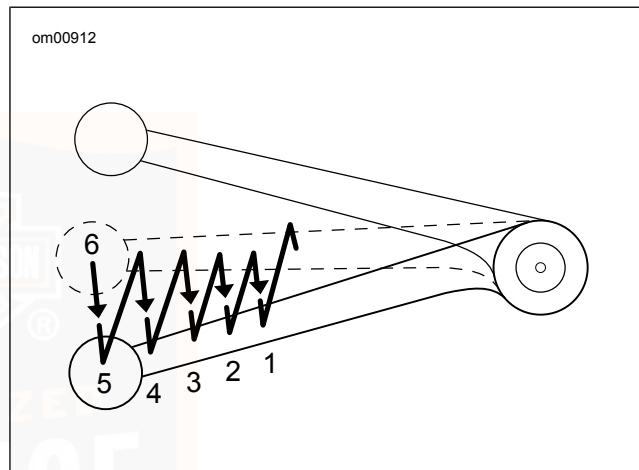
Abbildung 41. Schaltfolge: Herunterschalten GESCHWINDIGKEITSREGELUNG
