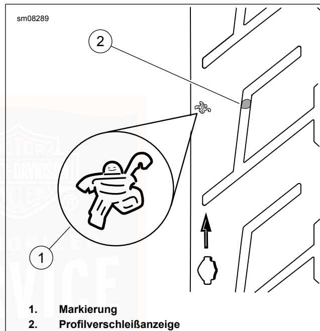
Abbildung 15. Profilverschleißanzeige: Michelin-Reifen
