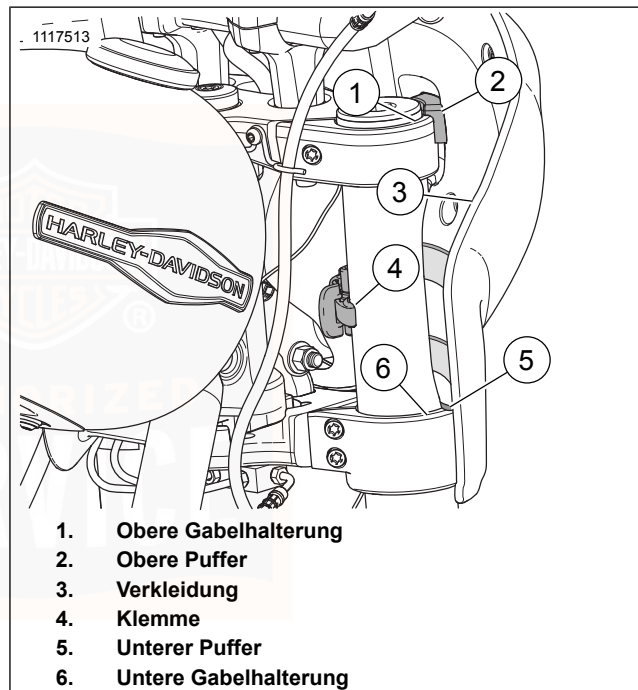
Abbildung 44. Eingebaute Verkleidung
