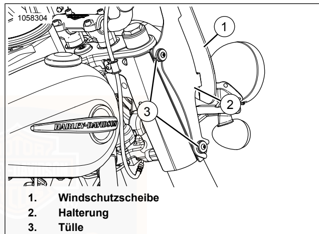
Abbildung 43. Windschutzscheiben-Baugruppe
