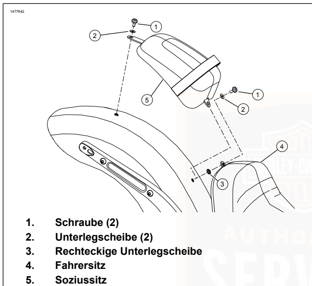
Abbildung 87. Zweiteilige Doppelsitzbank (Zwei Befestigungsteile)
