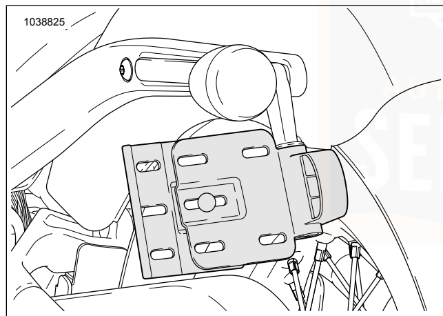
Abbildung 37. Seitlich befestigte Kennzeichenbaugruppe
