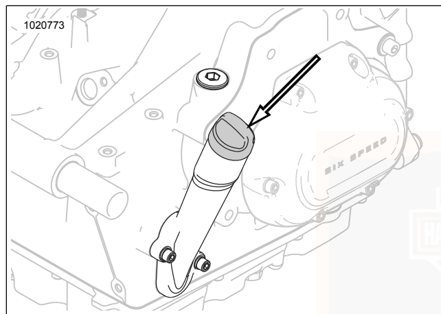
Abbildung 51. Motoröl-Einfüllverschlussstopfen
