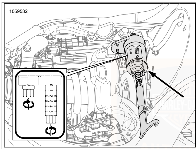
Abbildung 18. Vorspannungseinstellungsschraube
