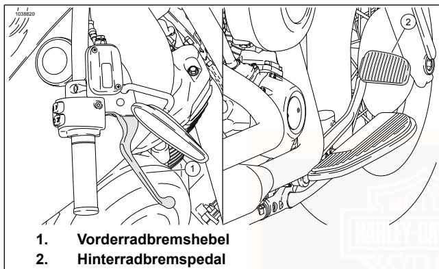
Abbildung 38. Bedienungselemente für Bremsen
