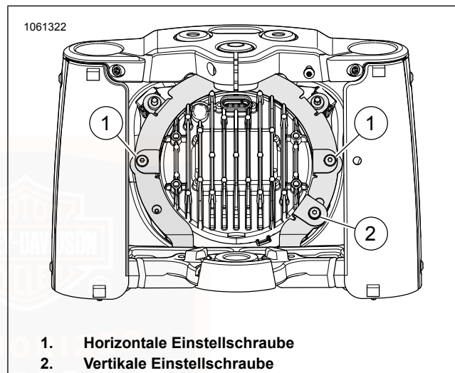
Abbildung 81. Scheinwerfereinstellung
