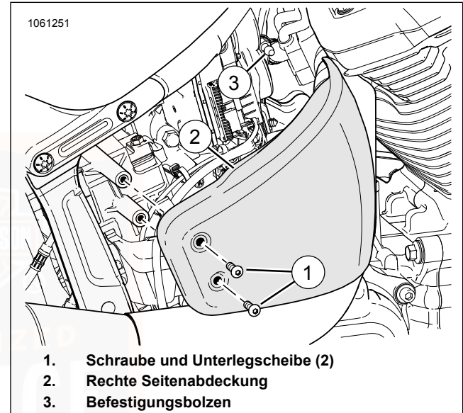
Abbildung 76. Rechte Seitenabdeckung
