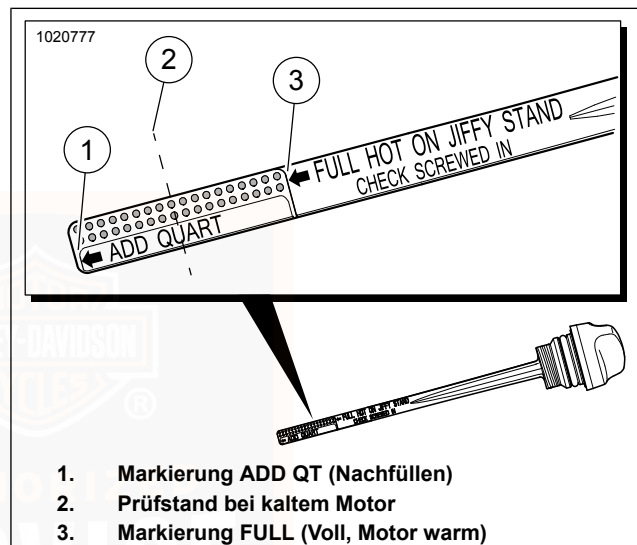
Abbildung 52. Motorölmesstab
