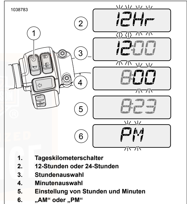
Abbildung 32. Zeitanzeigen
