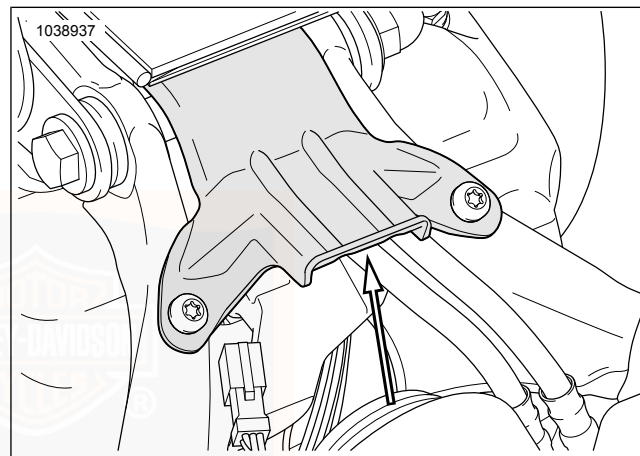
Abbildung 85. Sitzbefestigungshalterung
