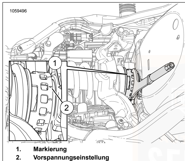
Abbildung 16. Vorspannungseinstellungsnocken
