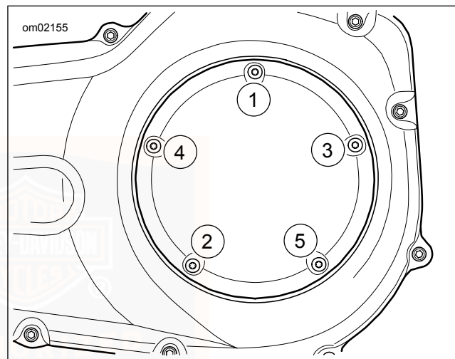
Abbildung 62. Anzugsreihenfolge für Kupplungsdeckel BREMSBELÄGE UND -SCHEIBEN PRÜFEN
