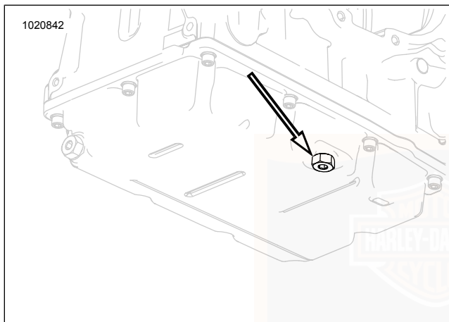
Abbildung 58. Getriebschmiermittelablassschraube PRIMÄRKETTENGESCHÄUSESCHMIERMittel WECHSELN
