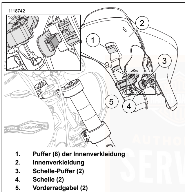
Abbildung 45. Verkleidungsklemmen
