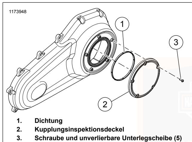
Abbildung 61. Kupplungsdeckel (Typisch)
