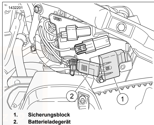
Abbildung 72. Sicherungen
